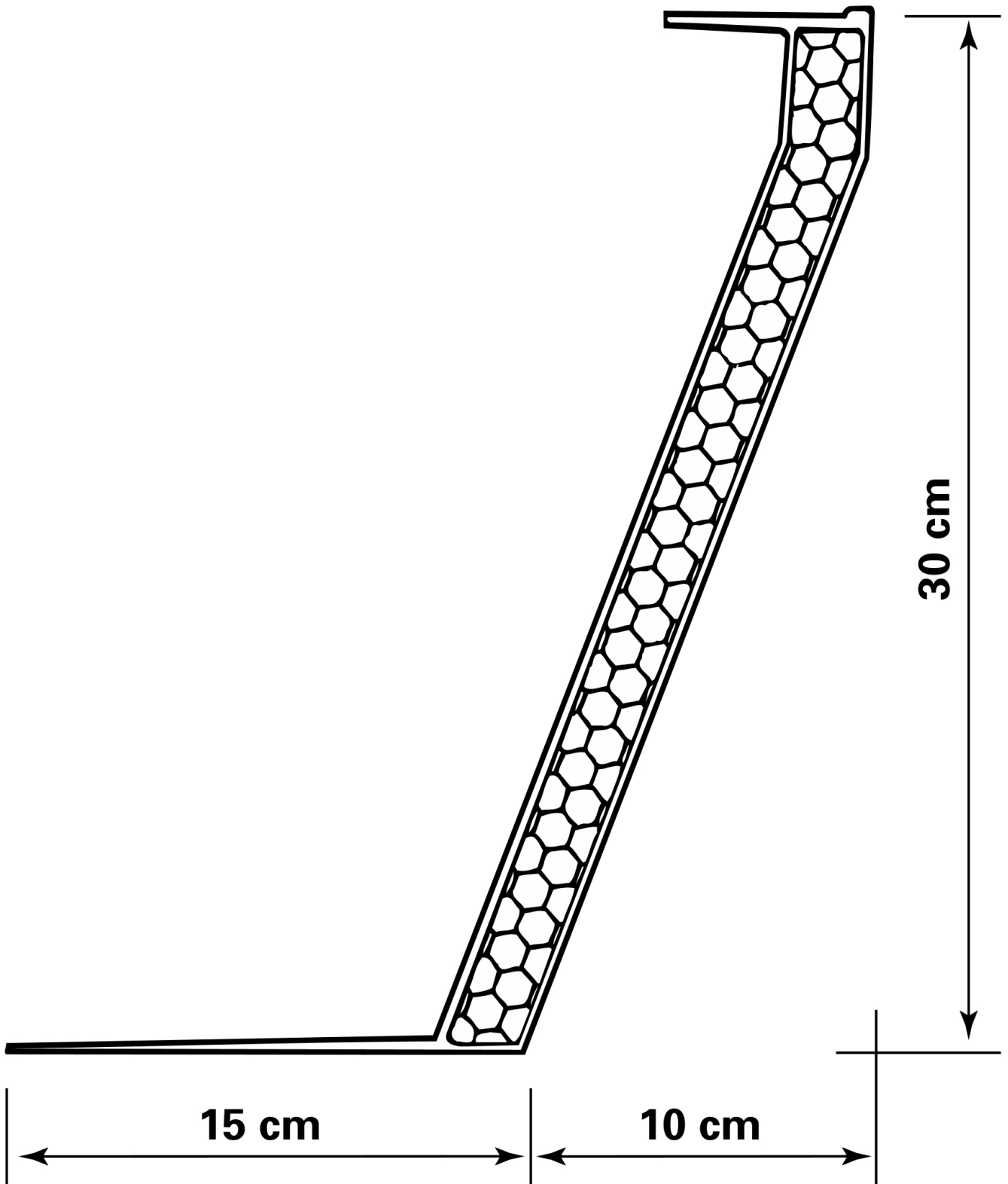
Detail SAVE2000 Polyester opstand type E30 / K=0,9
