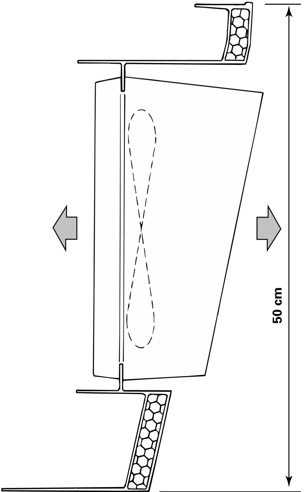
Detail SAVE2000 Polyester opstand met schroef ventilator
