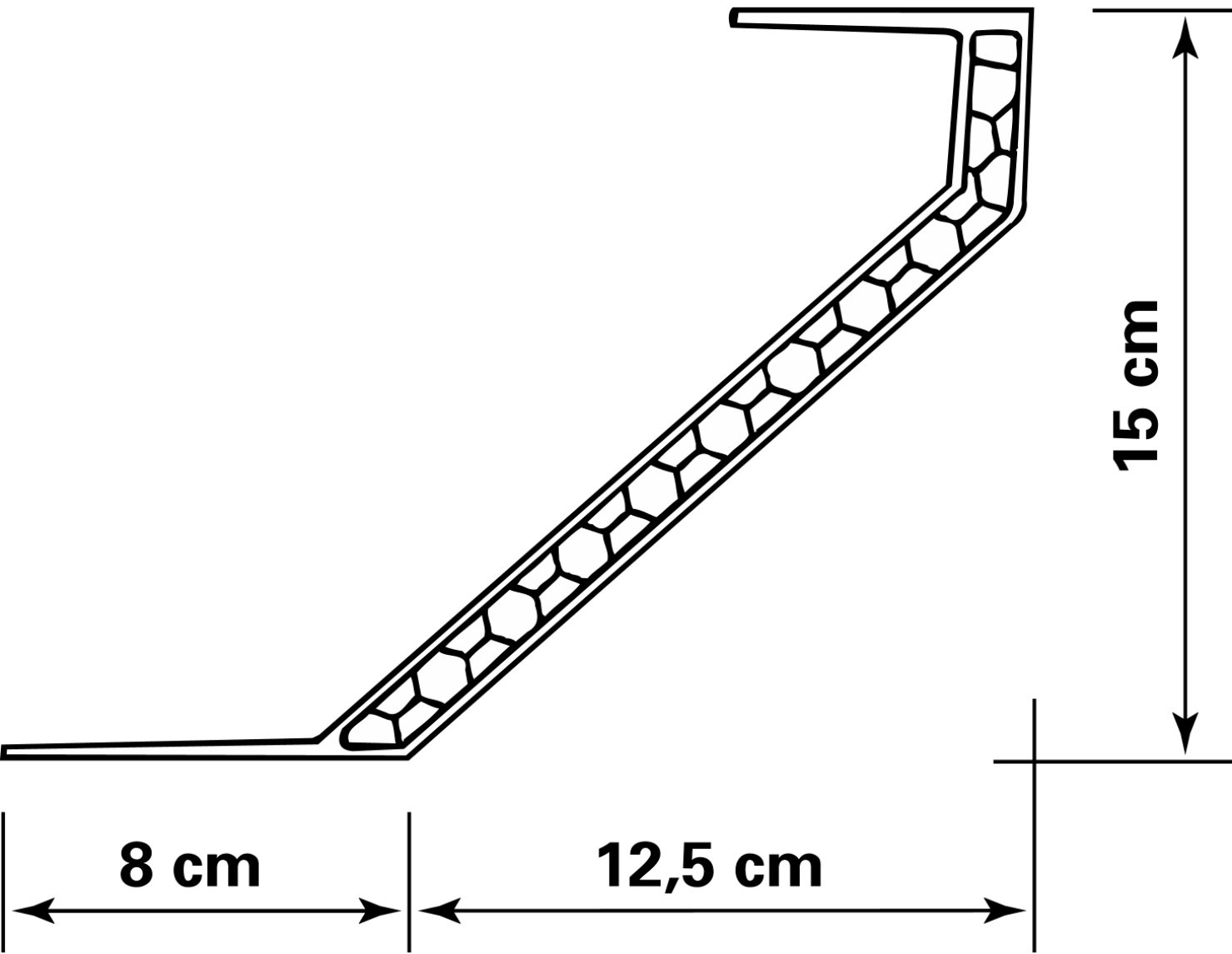
Detail SAVE2000 Polyester opstand type H 15 / K=1,6
