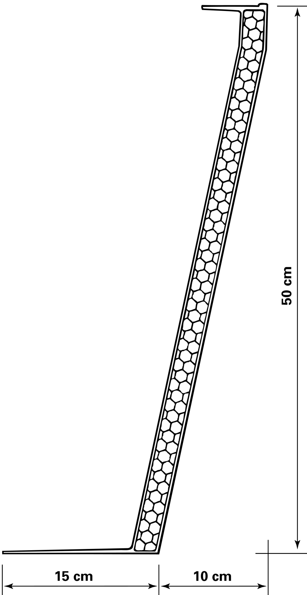
Detail SAVE2000 Polyester opstand type E50 / K=0,9
