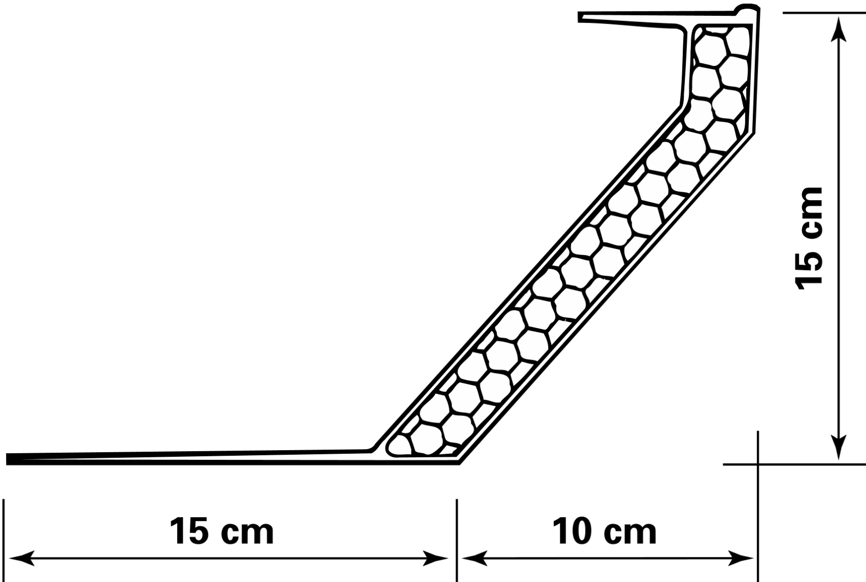
Detail SAVE2000 Polyester opstand type E15 / K= 0,9
