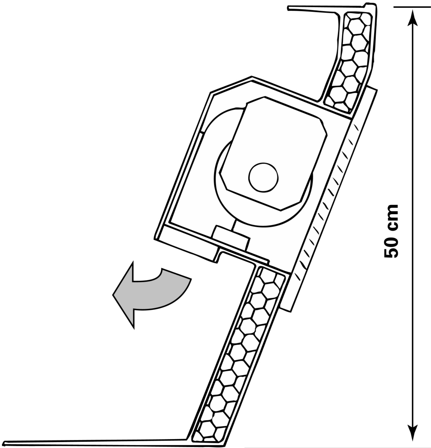
Detail SAVE2000 Polyester opstand met rolventilator
