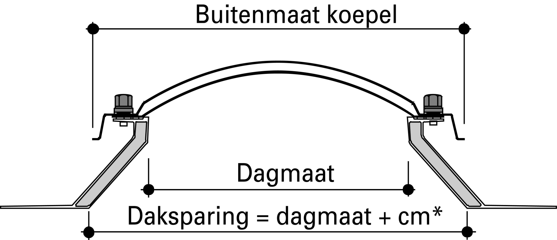
Doorsnede SAVE2000 opstand plus daglichtkoepel
