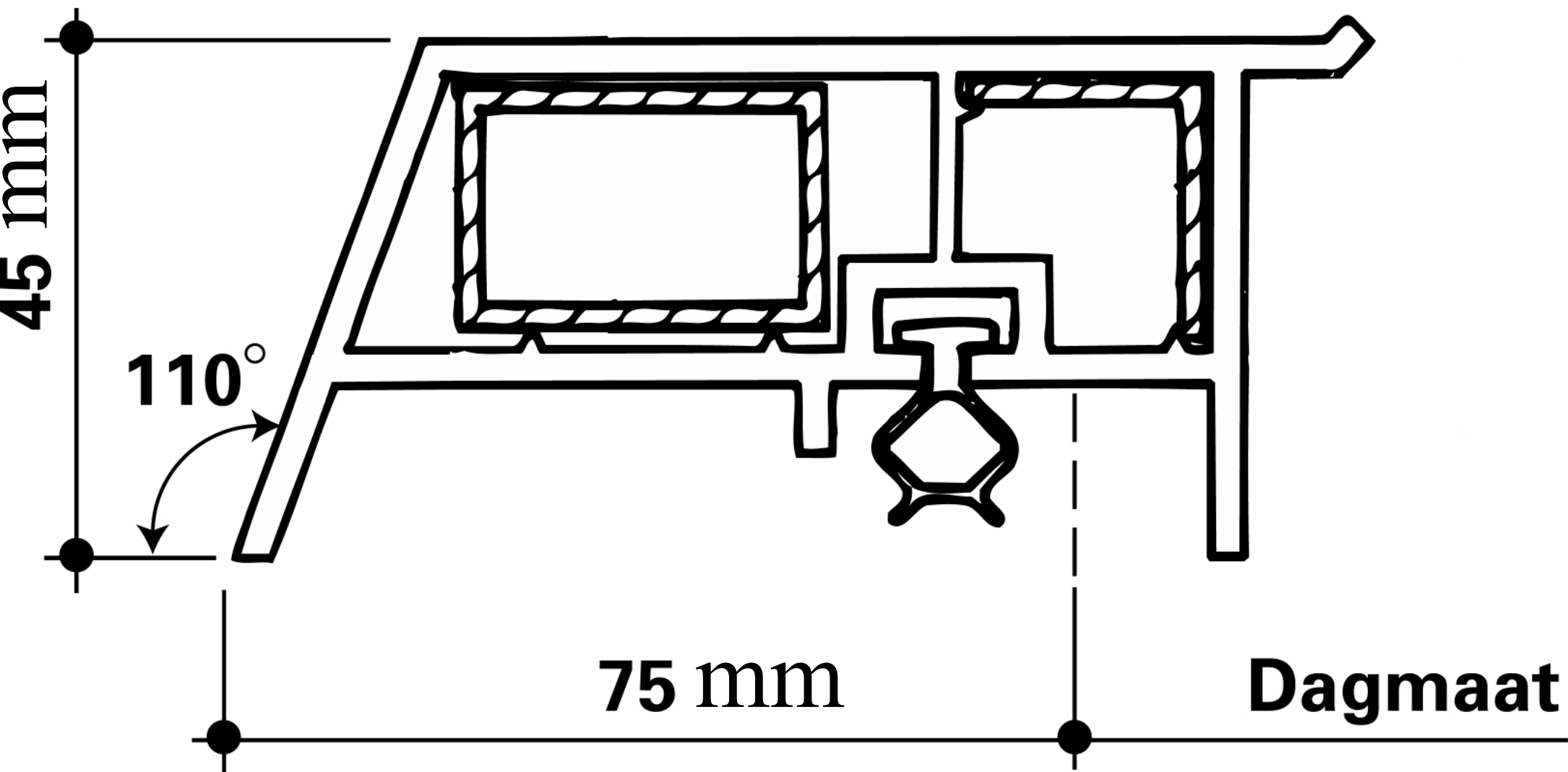
Detail SAVE2000 AVP ventilatieraam versterkt
